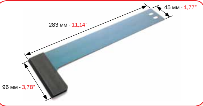
НОЖ ДЛЯ СНЯТИЯ МАРАШЕК: HICKEY REMOVER FOR: MITSUBISHI WEB OFFSET 11"
