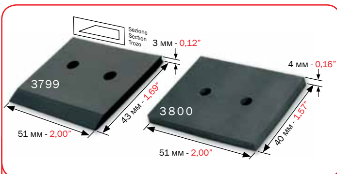
РАБОЧАЯ ЧАСТЬ НОЖА (РЕЗИНА) ДЛЯ СНЯТИЯ МАРАШЕК: RUBBER HICKEY REMOVER REPLACEMENT FOR: HEIDELBERG SPEEDMASTER 102-SORS/102CD
