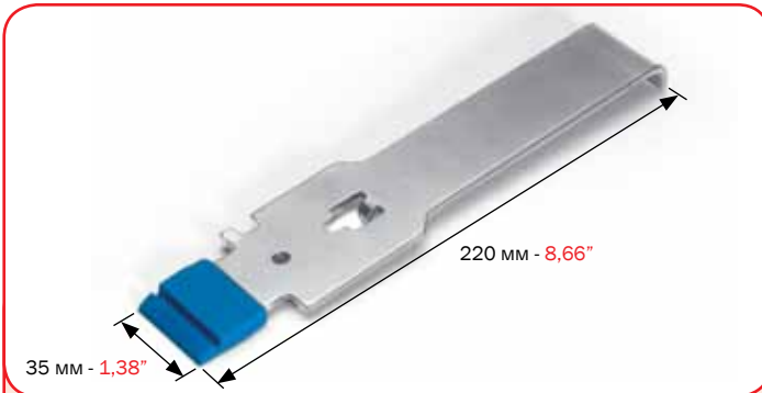
НОЖ ДЛЯ СНЯТИЯ МАРАШЕК В СБОРЕ ДЛЯ: COMPLETE HICKEY REMOVER FOR: HEIDELBERG SPEEDMASTER 74
