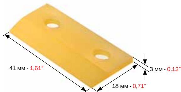
РАБОЧАЯ ЧАСТЬ НОЖА (РЕЗИНА) ДЛЯ СНЯТИЯ МАРАШЕК: RUBBER HICKEY REMOVER FOR: NEBIOLO COLORA 5000/7000
